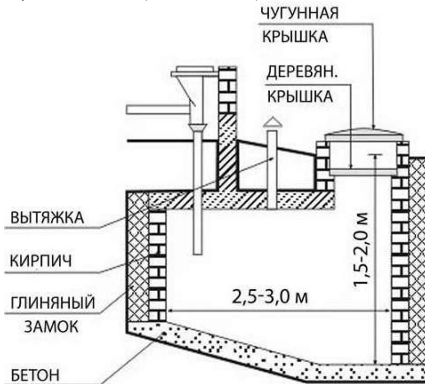
Рисунок 1 – Схема простейшей выгребной ямы из бетона
